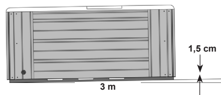
Pente de 1,5 cm par 3 m pour le bon écoulement de l'eau.
